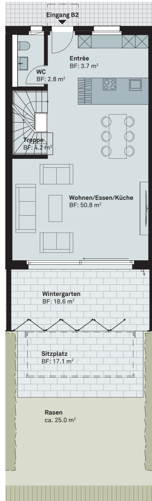
ERDGESCHOSS
